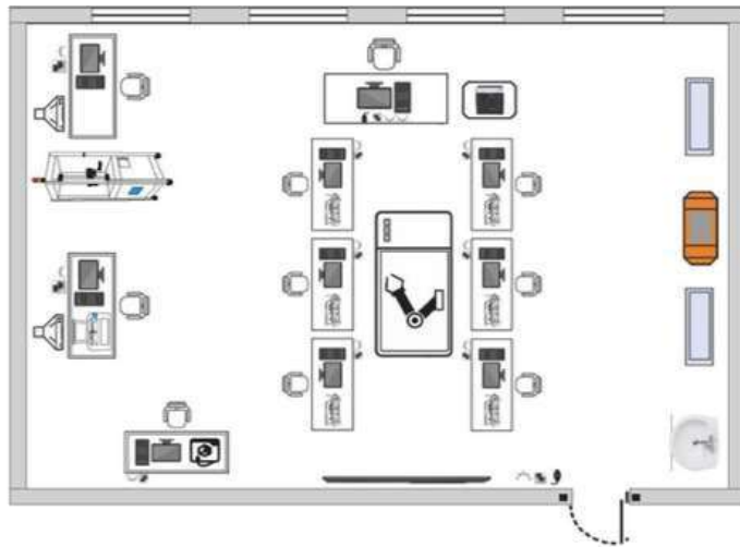
Рис. 5. Примерный план кабинет (количество рабочих мест определяет школа в зависимости от количества обучающихся в классе)
